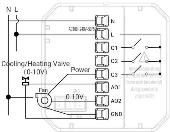
2-pipe, 0-10V valve, ECM fan
